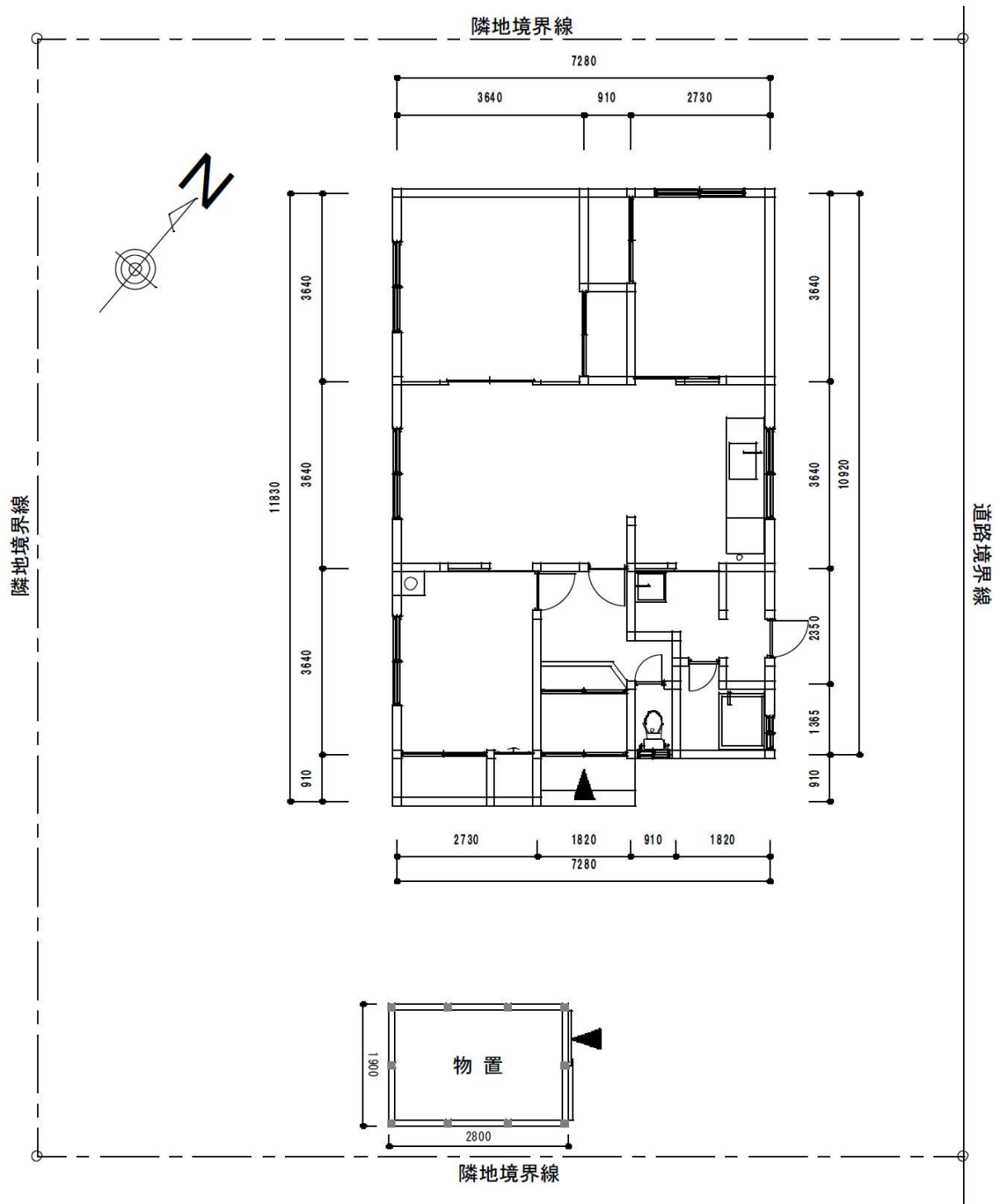
配置図
