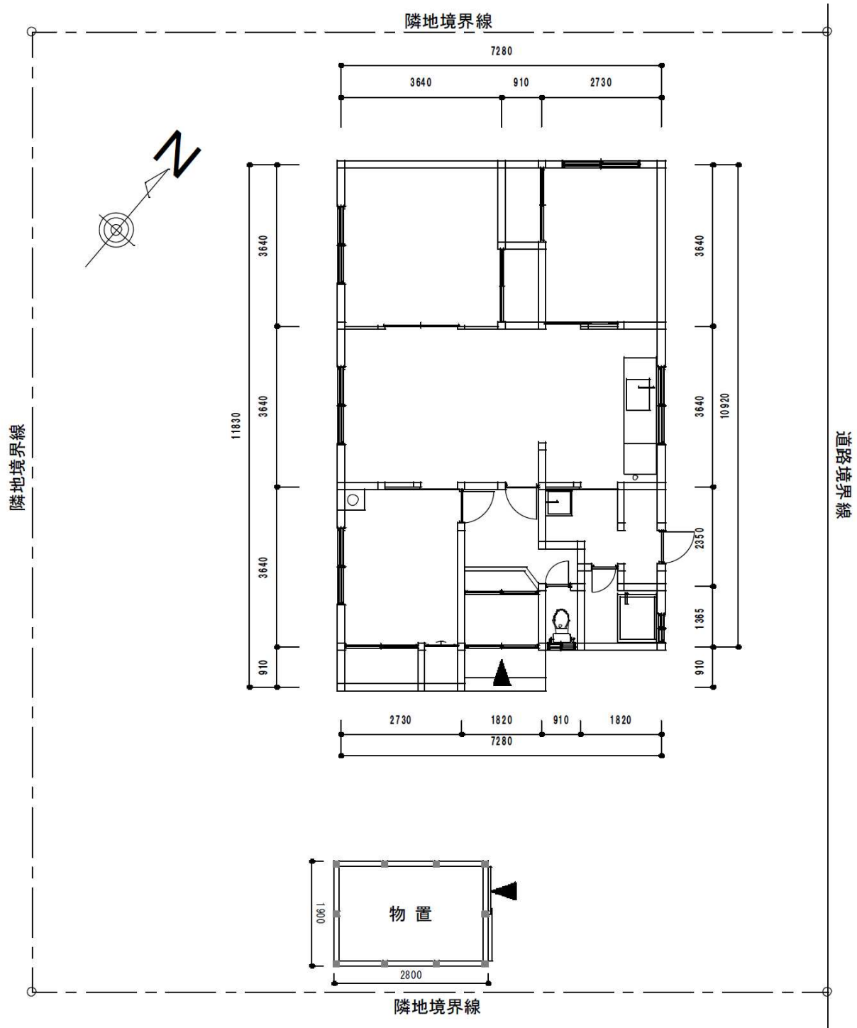
配置図
